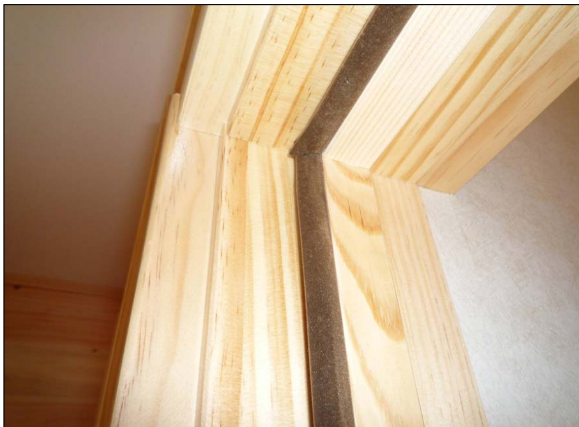
片開き(防音仕様) ピンチブロック取り付け状況 扉閉まっている状況
